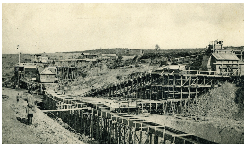
Слотки для подачи воды на промывку
